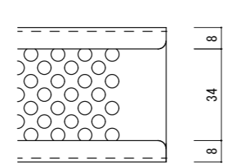
裏面詳細図
