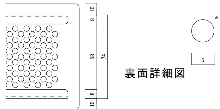
パンチング穴詳細図
